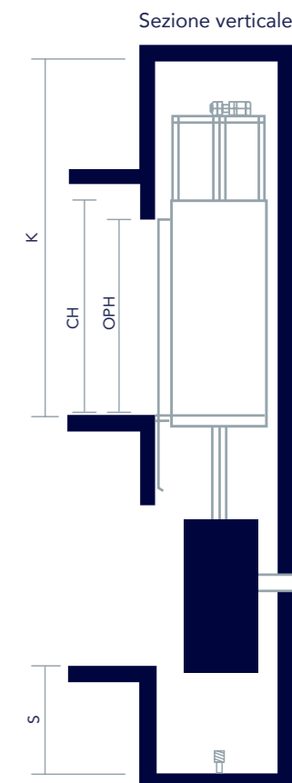
Un ingresso, porte telescopiche laterali
