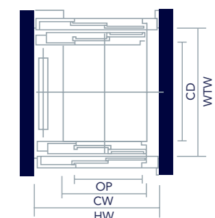
Due ingressi, porte telescopiche laterali
